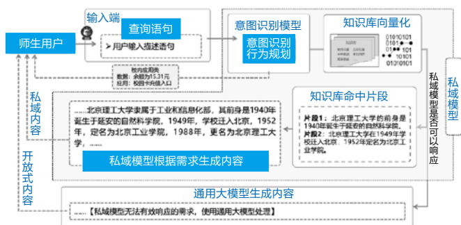
图2 “艾比特”交互流程
