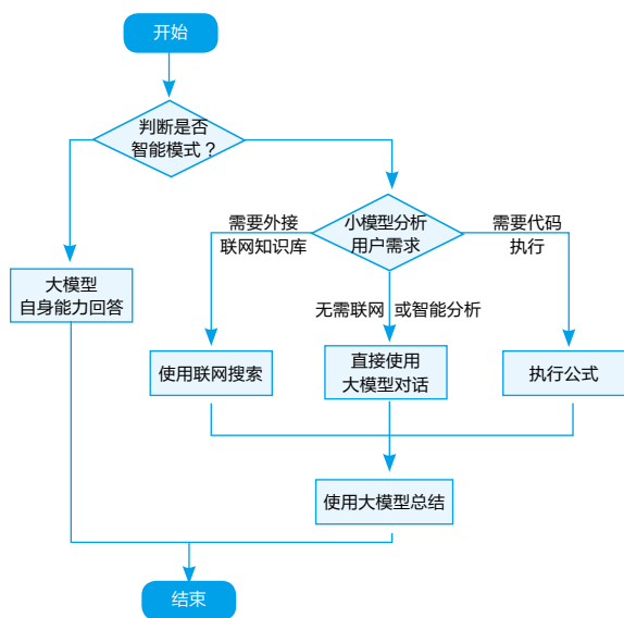
图 2 大模型应用中台流程设计
