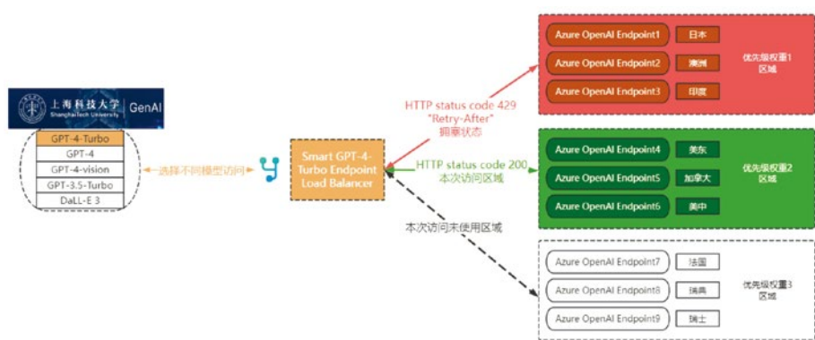
图2 智能负载均衡的逻辑
