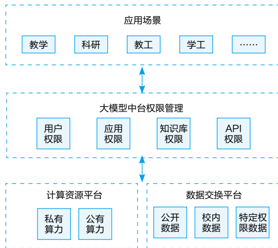
图 2 数据共享模式示意
