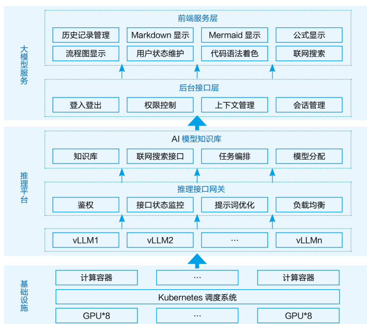
图 1 系统整体架构
