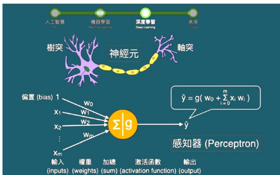
图4 神经网络模型示意
