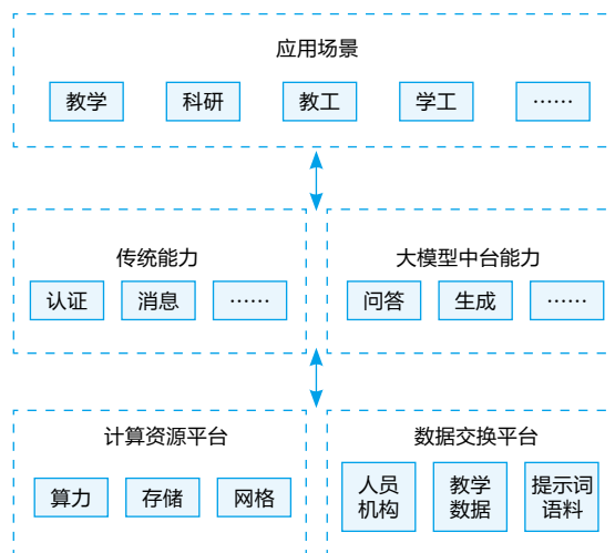
图 1 大模型中台架构示意图
