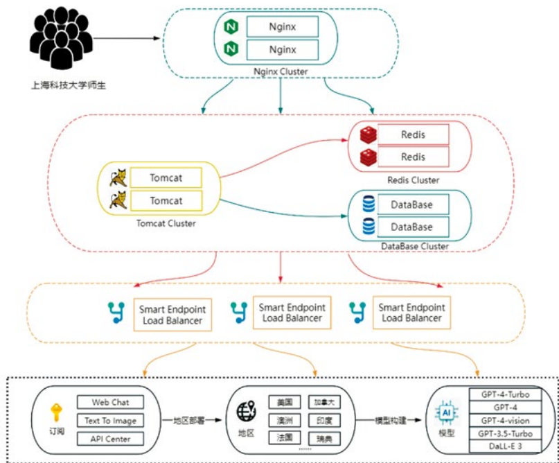
图 1 GenAI 业务架构
