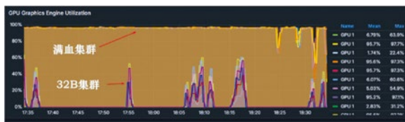
图 1 GPU 集群利用率动态分析: 32B 与满血集群性能对比
