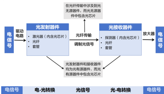
图8：光芯片工作原理
