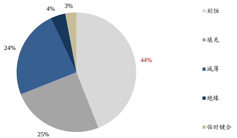
◆ 图34: 刻蚀是TSV工艺最大成本部分
