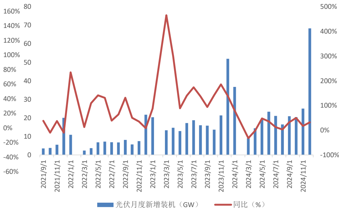
图表：国内光伏月度装机情况（GW）
