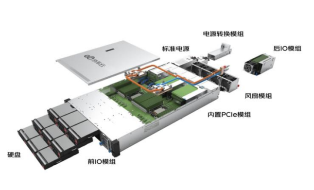
图42：京东云液冷服务器部署示意图
