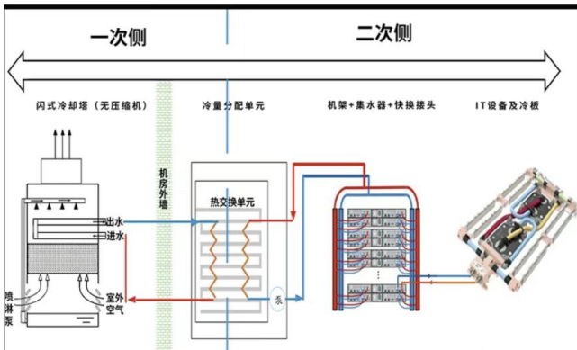
图43：冷板式液冷系统结构示意图
