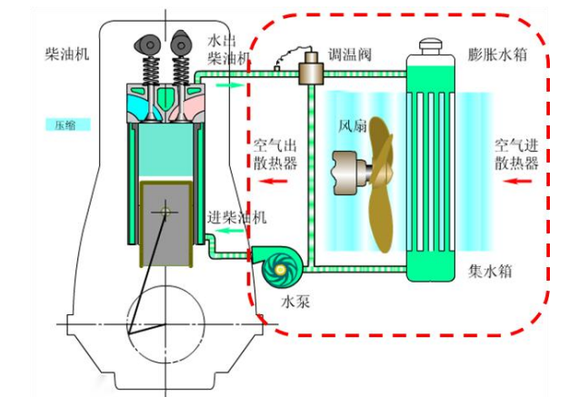
图18：柴油机冷却结构中，水的热量通过图右侧管壁和翅片高效地传递给空气
