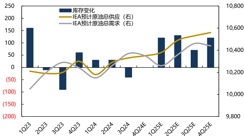
2024.11 IEA对全球原油供需及库存变化预测 (万桶/日)
