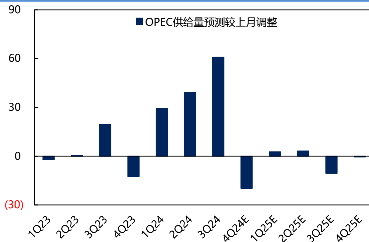
2024.11 OPEC对全球原油季度供给预测较2024.10调整 (万桶/日)
