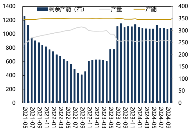
沙特产能、产量及剩余产能 (万桶/日, 万桶/日)
