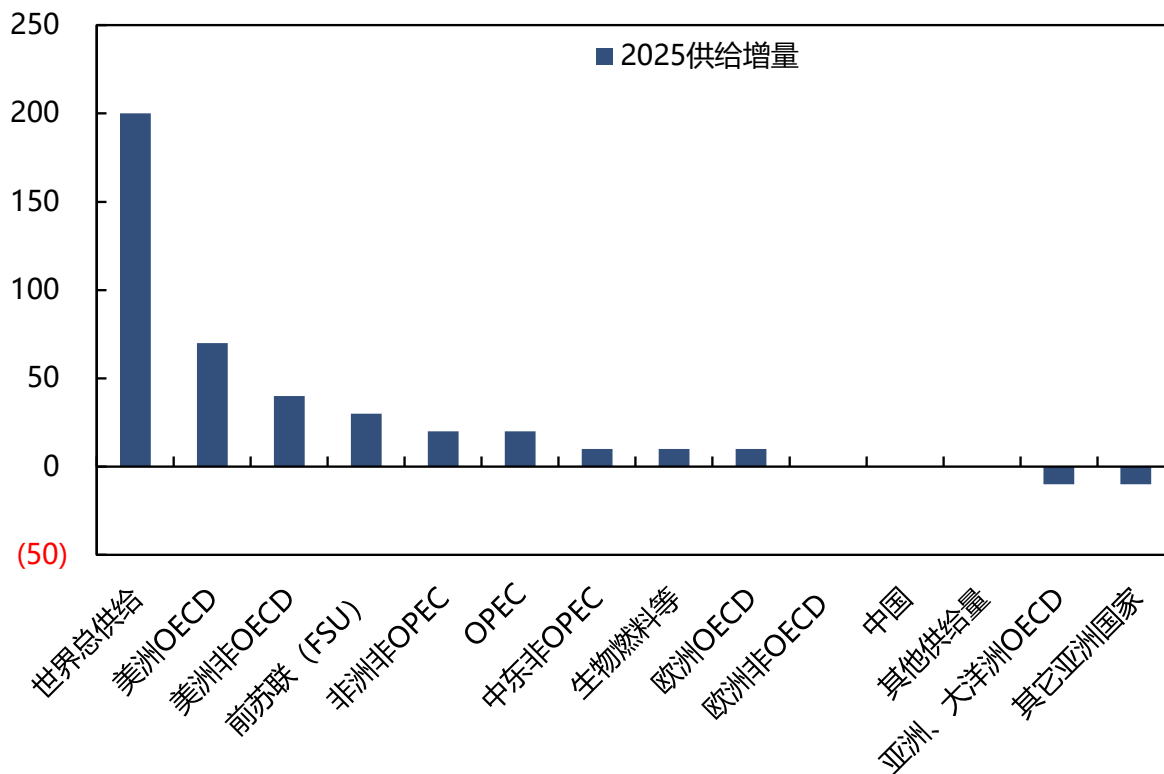
2024.11 IEA对2025年全球原油供给增量预测（万桶/日）
