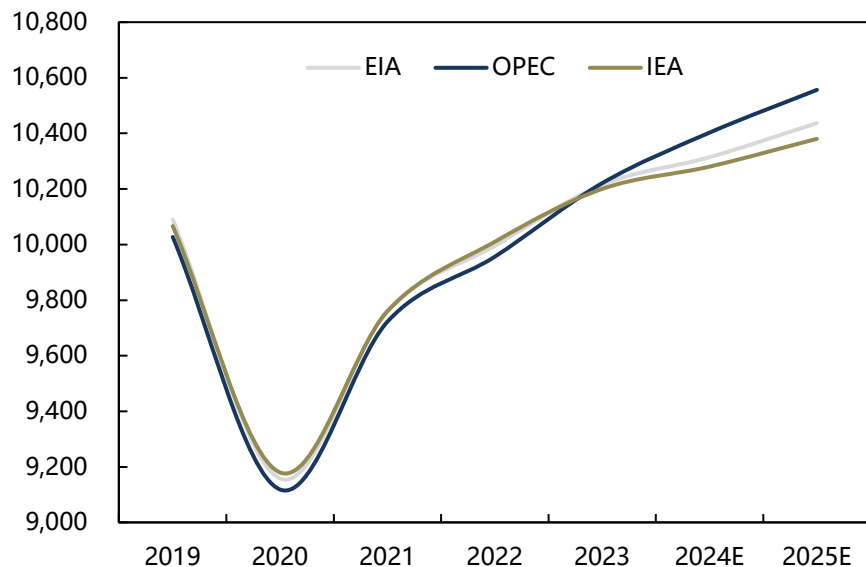
2024.11三大机构对全球原油年度需求预测量（万桶/日）
