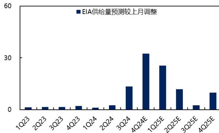
2024.11 EIA对全球原油季度供给预测较2024.10调整 (万桶/日)
