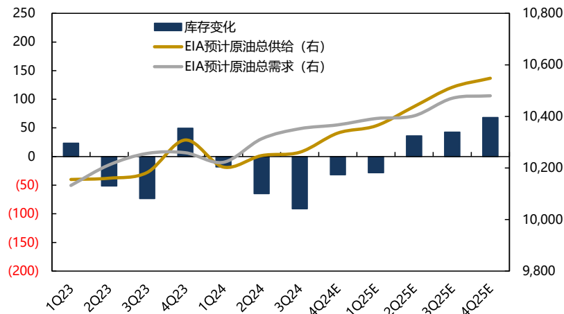
2024.11 EIA对全球原油供需及库存变化预测 (万桶/日)
