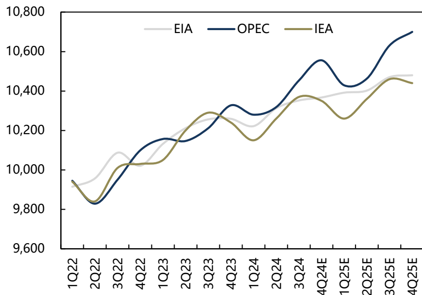
2024.11三大机构对全球原油季度需求预测量 (万桶/日)
