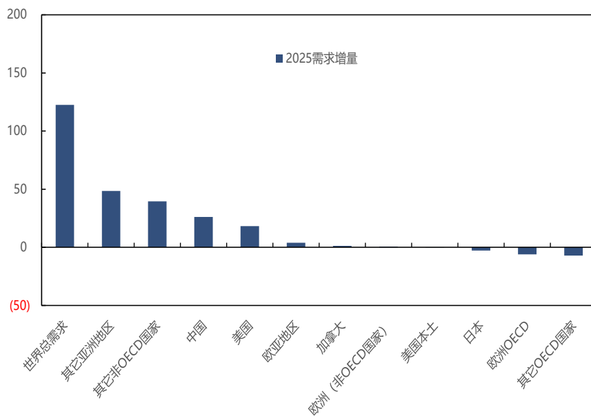
2024.11 EIA预测2025年全球原油分地区需求增量（万桶/日）
