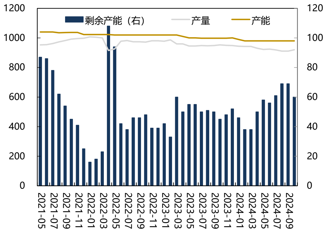
俄罗斯原油产能、产量（万桶/日，万桶/日）
