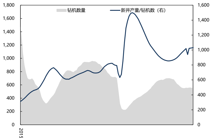
美国七大页岩油产区总钻机数量和平均单个钻机对应的新井原油产量（台，桶/日）
