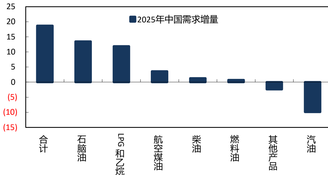
2024.11 IEA预测2025中国原油分产品需求增量（万桶/日）
