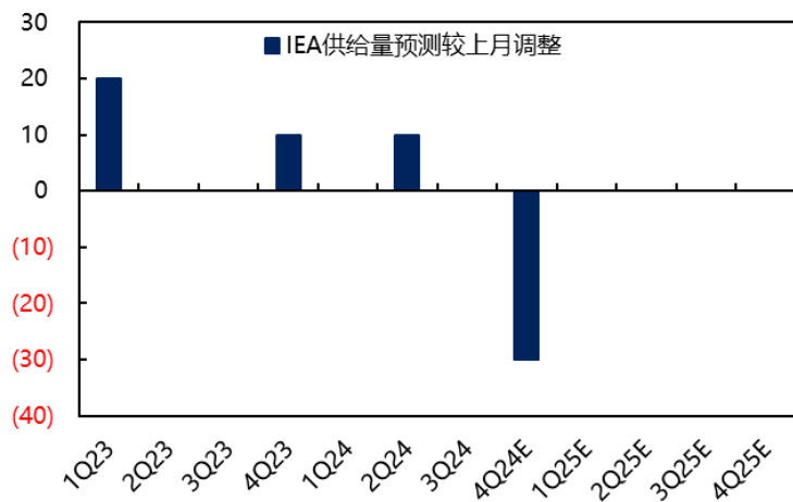
2024.11 IEA对全球原油季度供给预测较2024.10调整 (万桶/日)
