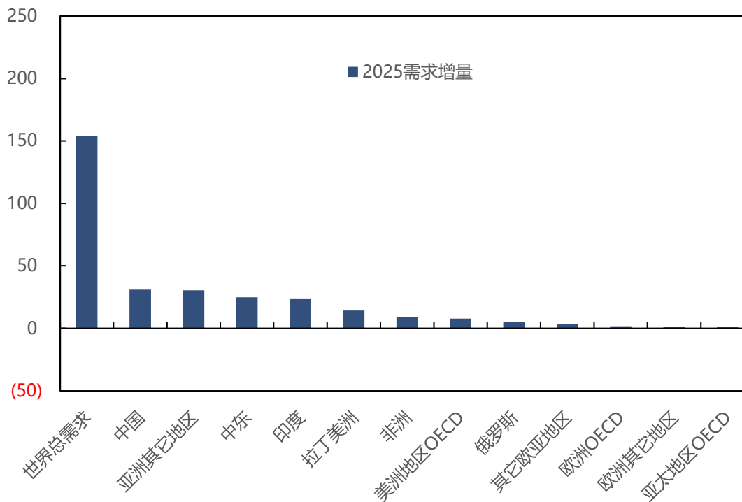
2024.11 OPEC预测2025年全球原油分地区需求增量 (万桶/日)
