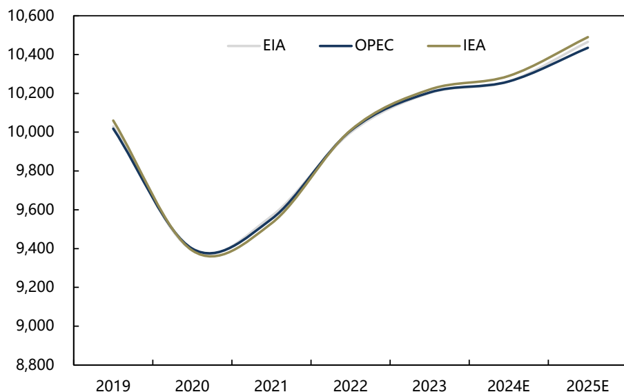
2024.11 三大机构对全球原油年度供给预测量（万桶/日）
