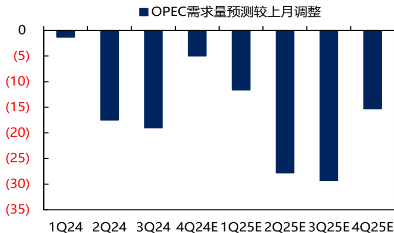
2024.11 OPEC对全球原油季度需求预测较2024.10调整 (万桶/日)
