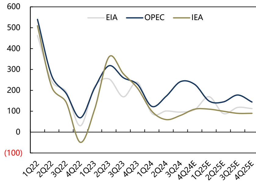
2024.11三大机构对全球原油季度需求预测同比增量 (万桶/日)
