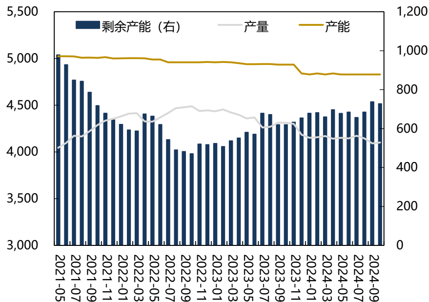
OPEC+产能、产量及剩余产能（万桶/日，万桶/日）
