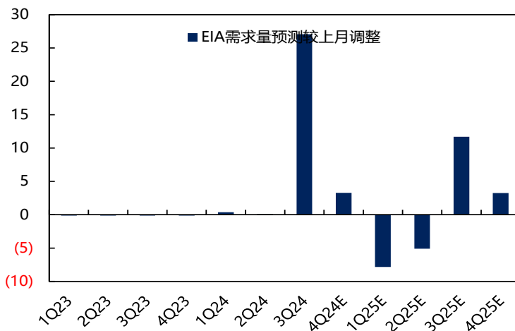
2024.11 EIA对全球原油季度需求预测较2024.10调整 (万桶/日)
