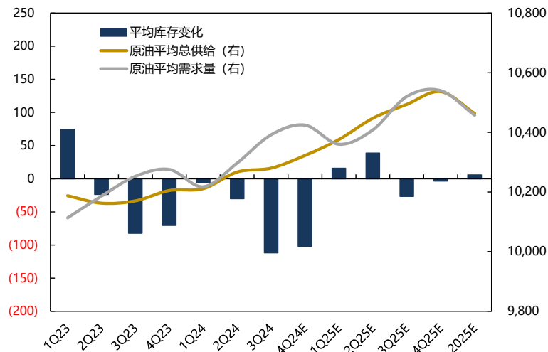
2024.11 三大机构对全球原油供需及库存变化预测均值 (万桶/日)
