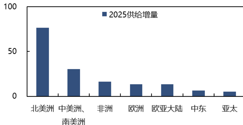
2024.11 EIA对2025年非OPEC原油供给增量预测 (万桶/日)
