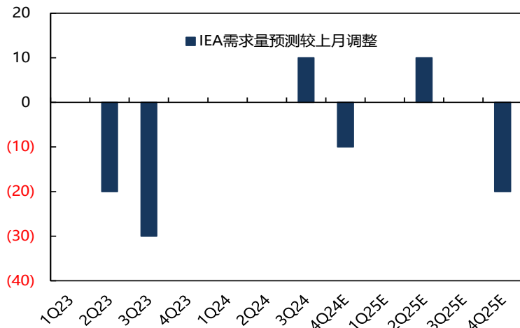
2024.11 IEA对全球原油季度需求预测较2024.10调整 (万桶/日)
