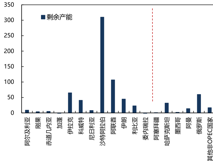
IEA对OPEC+2024.11的剩余产能测算（万桶/日）
