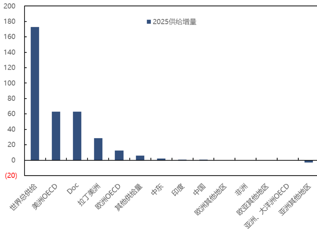
2024.11 OPEC对2025年全球原油供给增量预测（万桶/日）
