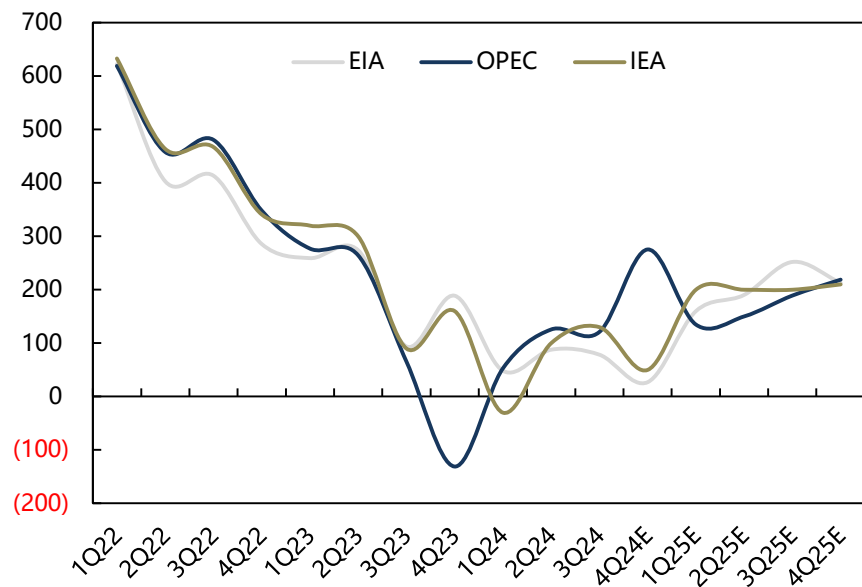
2024.11 三大机构对全球原油季度供给预测同比增量（万桶/日）
