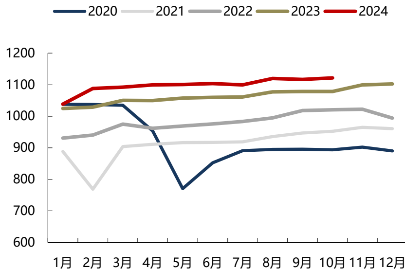
Lower 48 States (excl GOM) 产量 (万桶/日)
