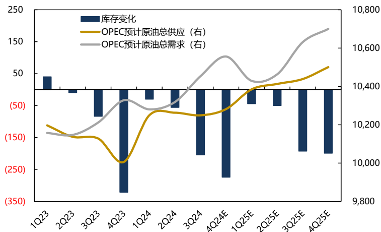
2024.11 OPEC对全球原油供需及库存变化预测 (万桶/日)
