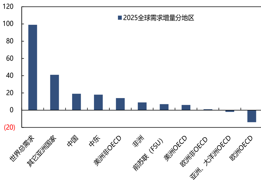
2024.11 IEA预测2025全球原油分地区需求增量（万桶/日）
