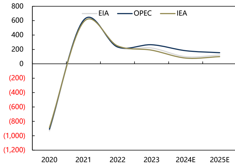
2024.11三大机构对全球原油年度需求预测同比增量（万桶/日）
