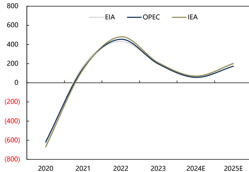
2024.11 三大机构对全球原油年度供给预测同比增量（万桶/日）
