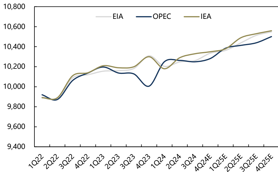
2024.11三大机构对全球原油季度供给预测量（万桶/日）
