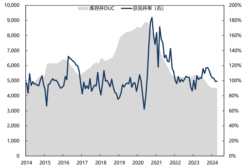
美国页岩油库存井和总完井率（口，%）
