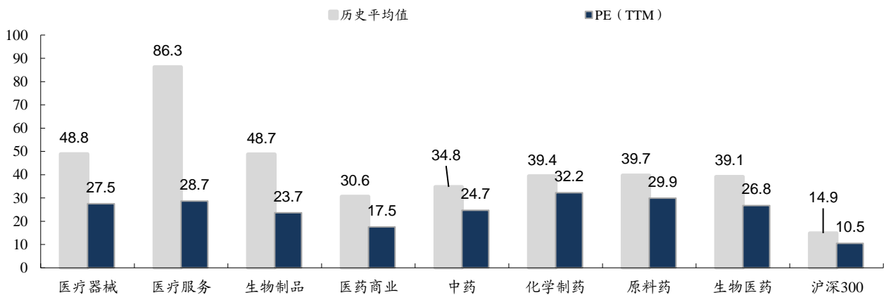
图15: 医药板块估值情况
