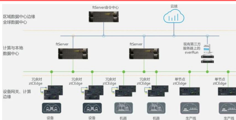
图 20：边缘计算与智能制造（物联网）融合典型样例
