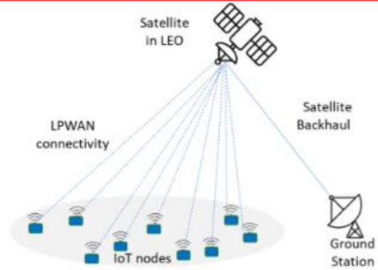
图 24：IoT 通信连接架构概览(DtS-IoT)
