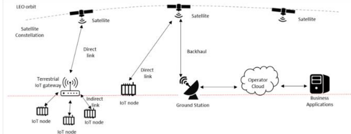
图 22：卫星物联网的物理架构显示
