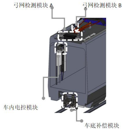
图 92 本方案核心硬件产品
