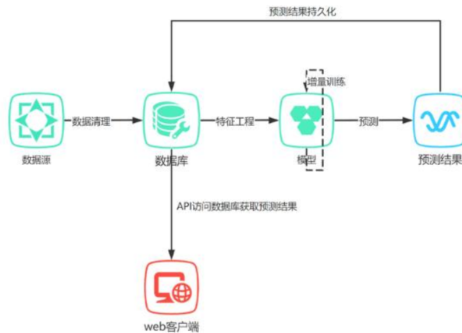
图 78 数据处理流程
