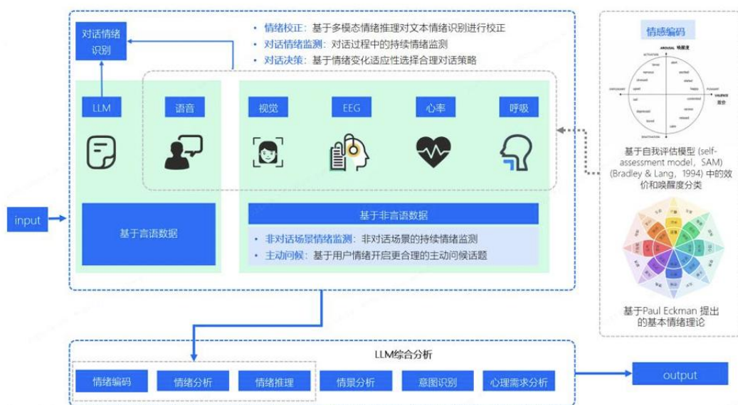
图 20 基于多模态的情感计算方案
