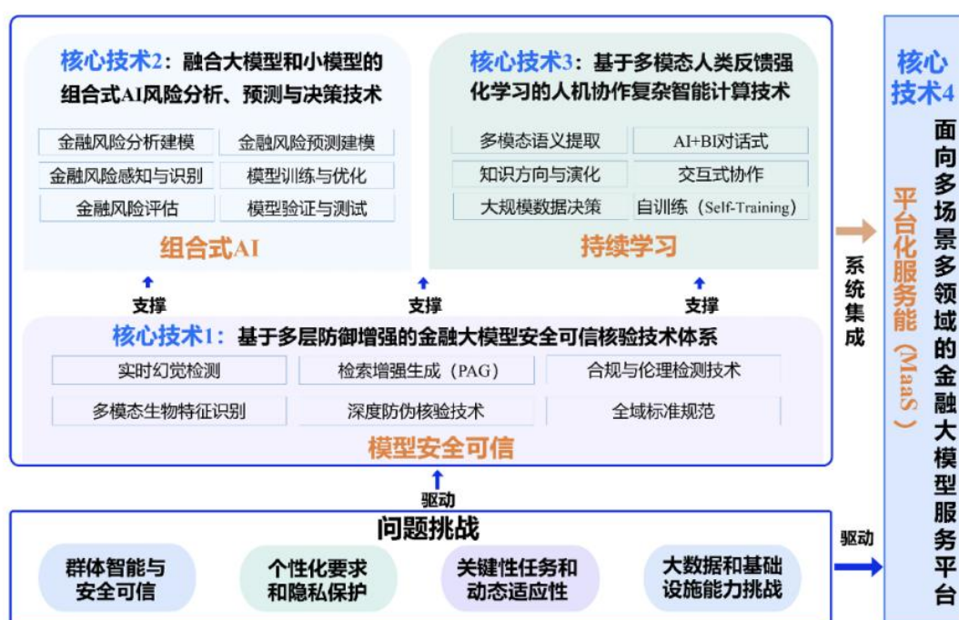
图 69 金融大模型技术架构图
