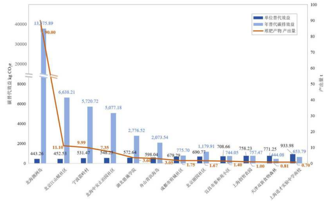
图 4-21 各项目腐殖酸替代碳排效益
