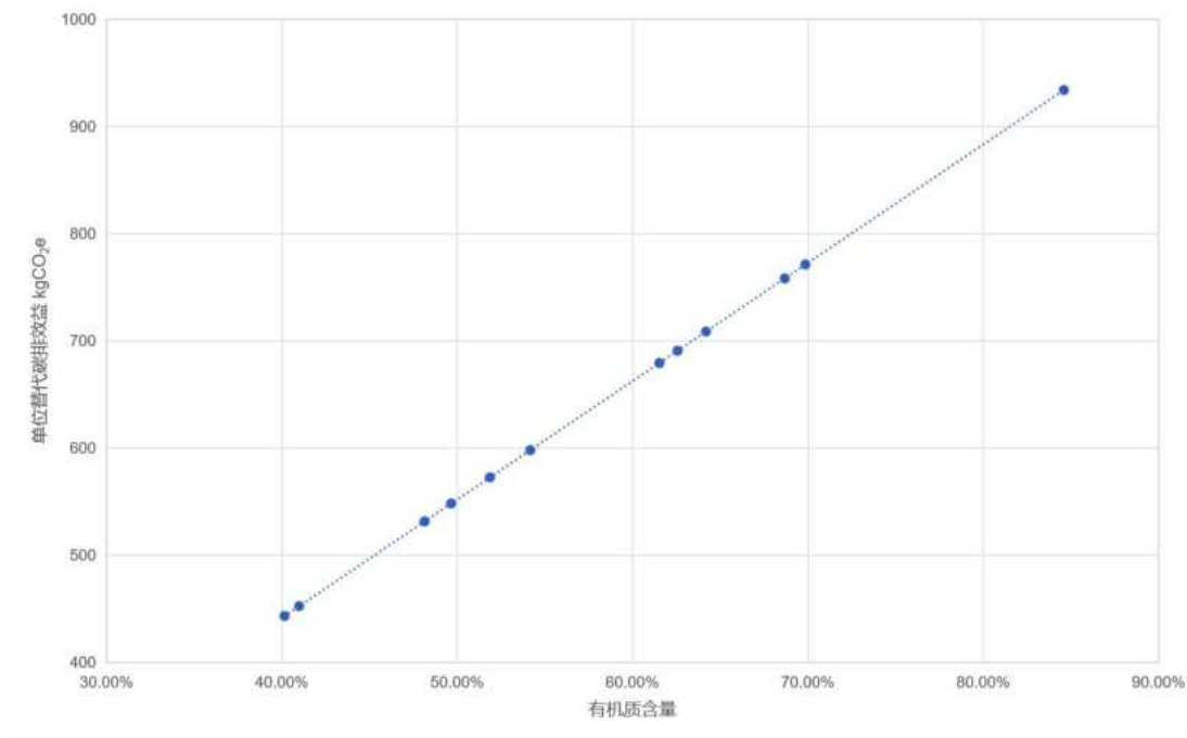
图 4-20 有机质含量和单位替代碳排效益关系
