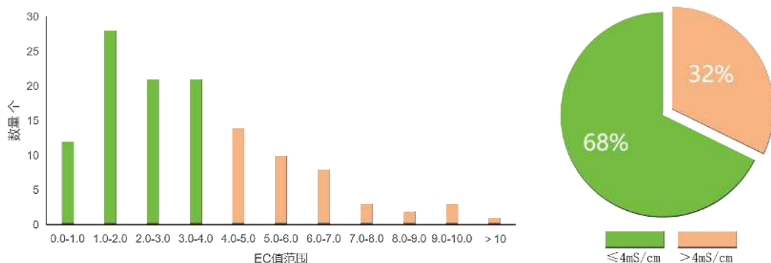
图 3-8 平台堆肥产物样品 EC 值不同区间数量及占比统计
