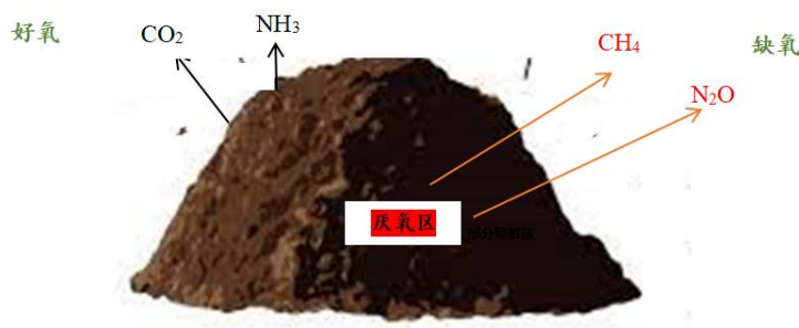
图 4-3 堆肥过程中主要排放的温室气体
