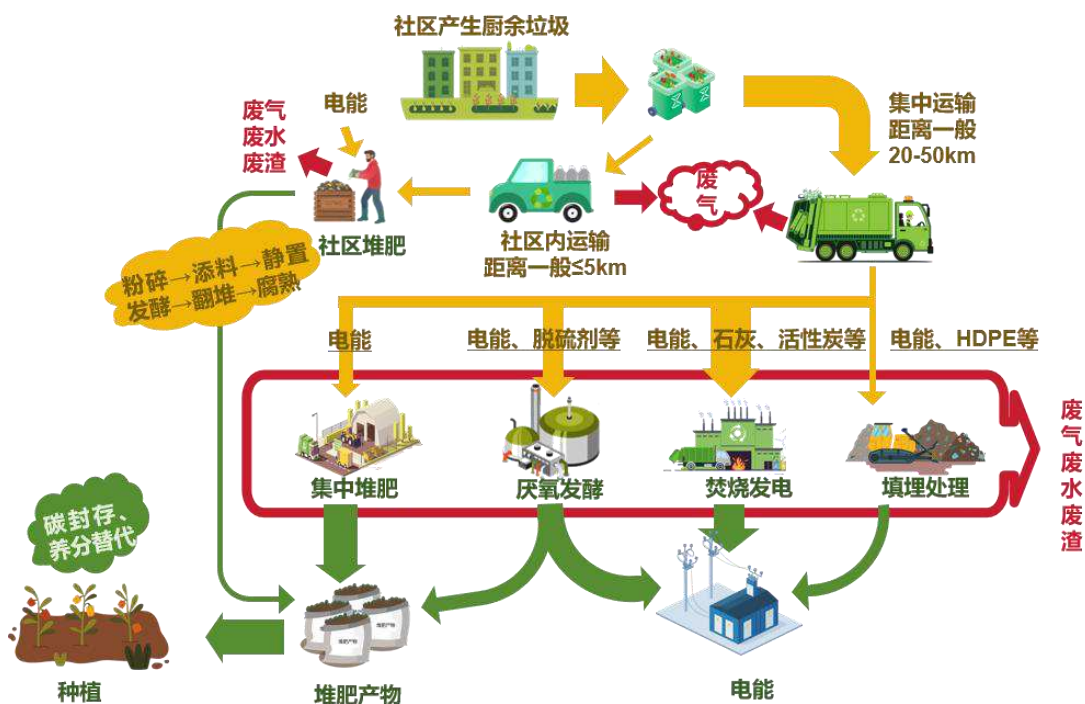
图 2-2 社区堆肥与传统处理方式系统边界
