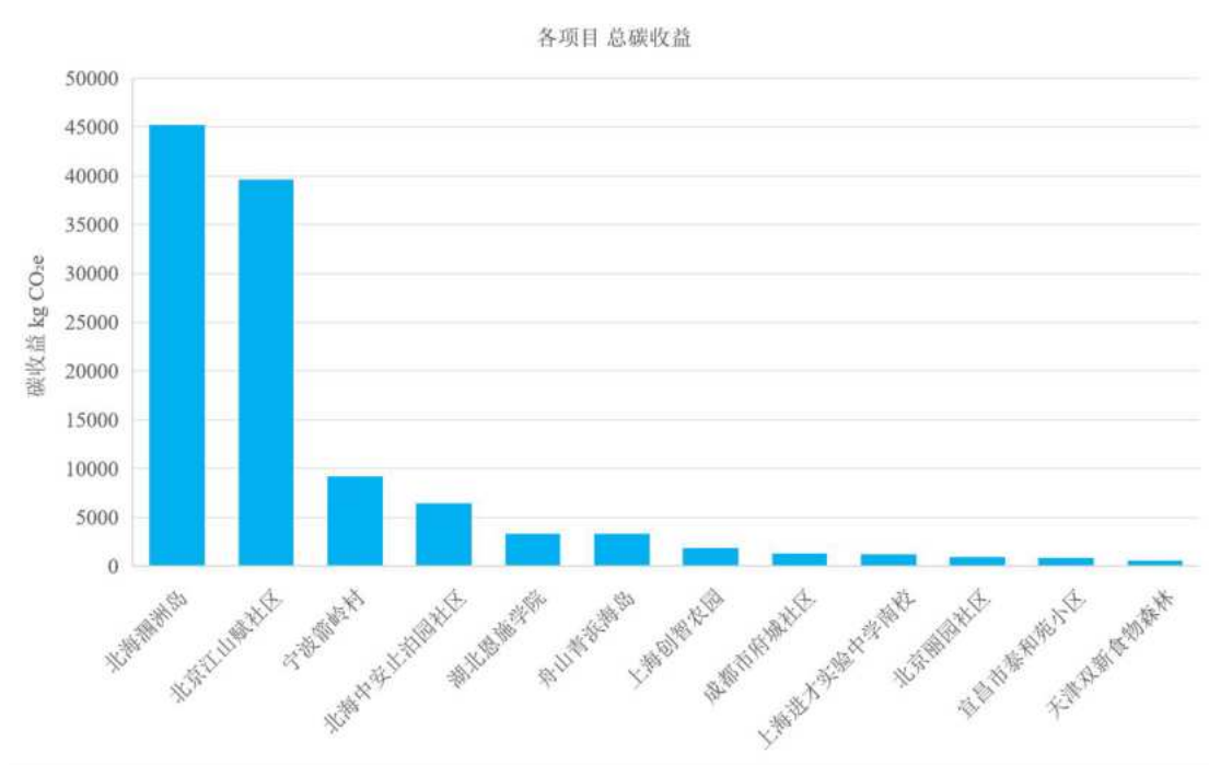
图 4-22 社区堆肥各项目堆肥碳收益
