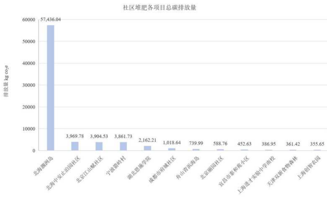
图 4-14 社区堆肥各项目堆肥总碳排放量
